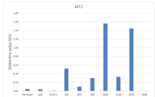
Slika 9 Grafički prikaz rezultata mjerenja u MT.2
