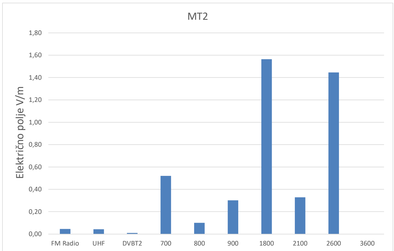
Slika 14 Cijeli radiofrekvencijski spektar
