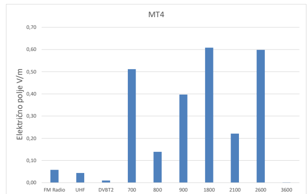
Slika 11 Grafički prikaz rezultata mjerenja u MT.4
