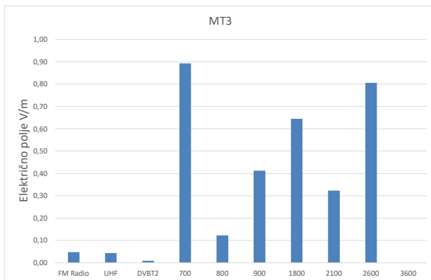
Slika 10 Grafički prikaz rezultata mjerenja u MT.3
