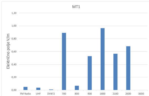
Slika 8 Grafički prikaz rezultata mjerenja u MT.1
