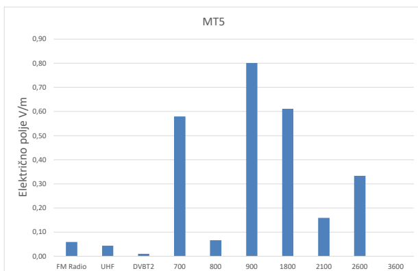
Slika 12 Grafički prikaz rezultata mjerenja u MT.5
