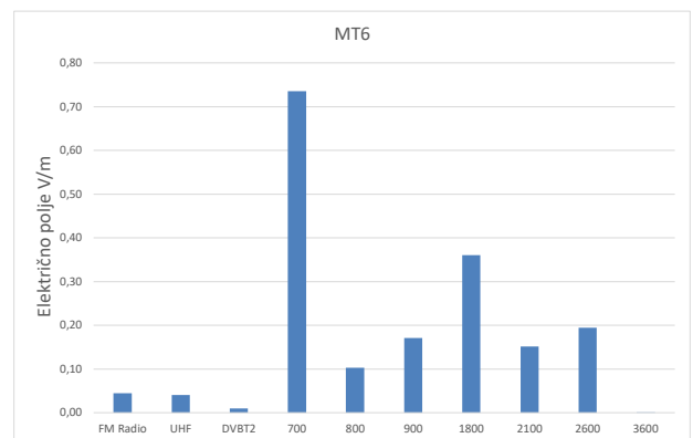
Slika 13 Grafički prikaz rezultata mjerenja u MT.6
